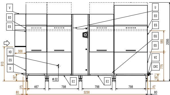
Zij aanzicht
